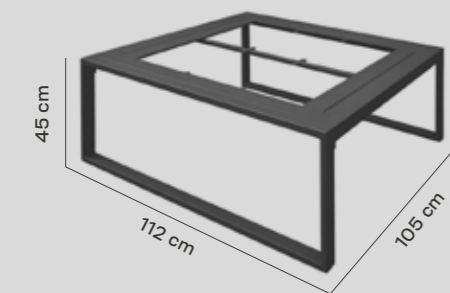
ESTRUCTURA MESA 105 X 112 X 45 CM
