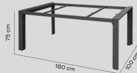
ESTRUCTURA MESA 180 X 100 X 75 CM
